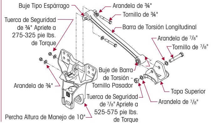
FIGURA 6-4 Tornillería del Paquete de Sujeción
