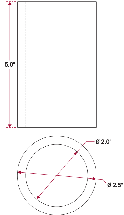
HERRAMIENTA DE RECIBO Para Bujes de Barra de Torsión
