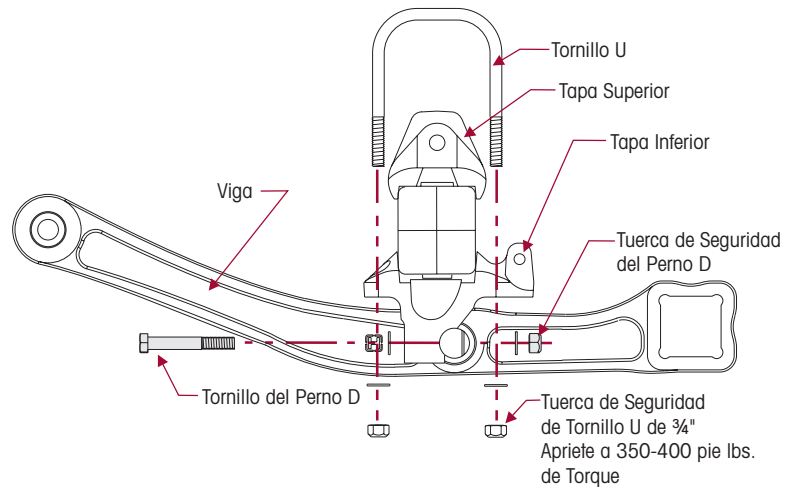
FIGURA 6-4 Tornillería del Paquete de Sujeción
