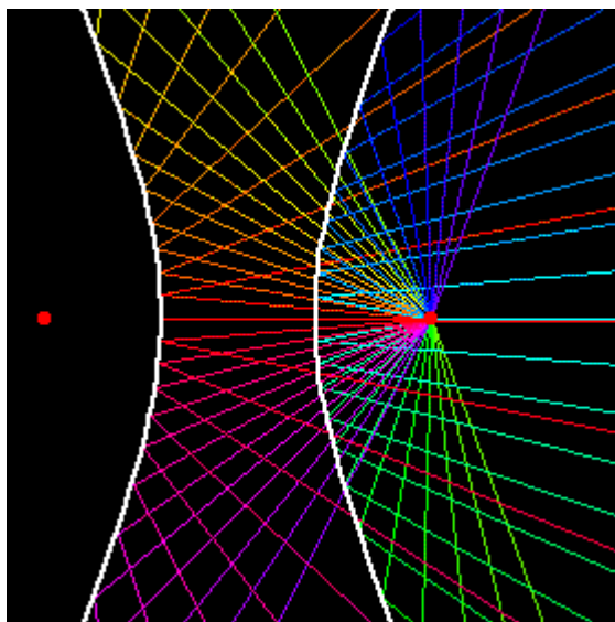
Fig.1 Proprietà ottica dell' iperbole
