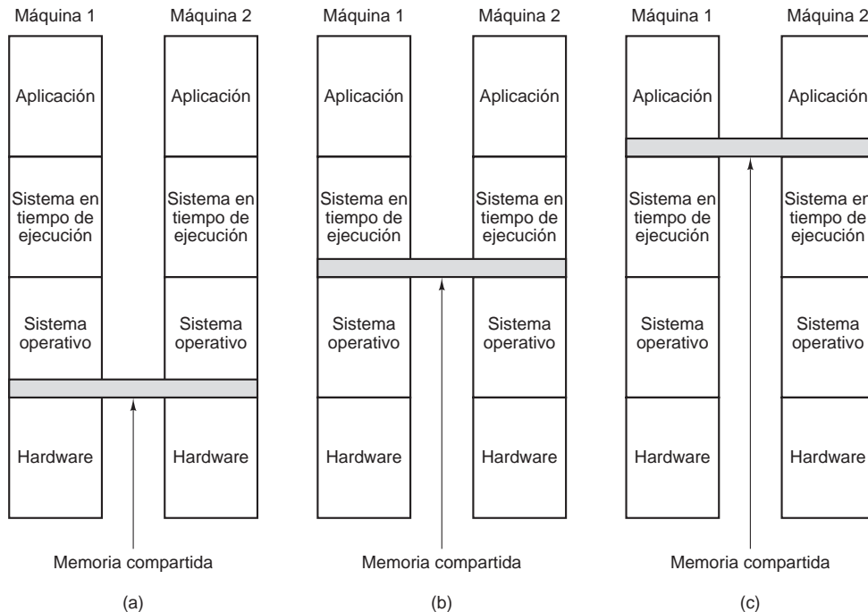
Figura 8-21. Varios niveles en donde se puede implementar la memoria compartida. (a) El hardware. (b) El sistema operativo. (c) Software a nivel de usuario.
