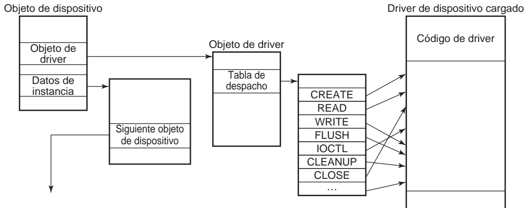
Figura 11-38. Un nivel individual en una pila de dispositivos.
