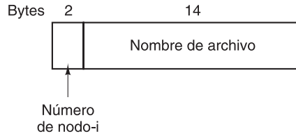
Figura 4-33. Una entrada de directorio de UNIX V7.
