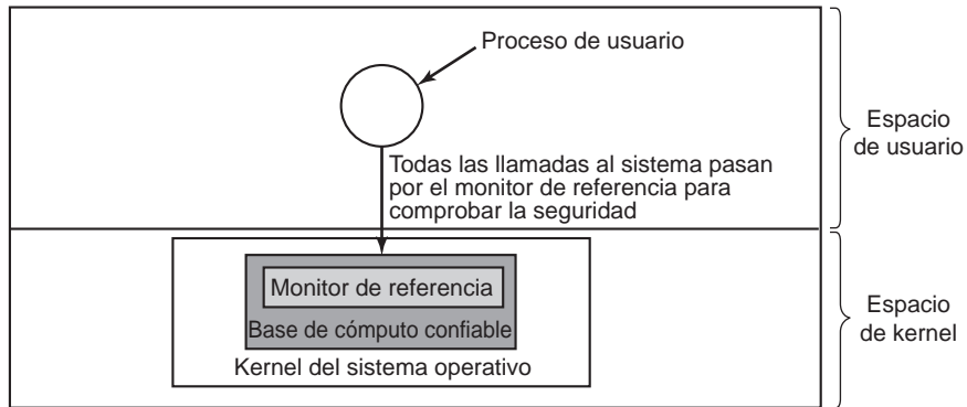
Figura 9-11. Un monitor de referencia.
