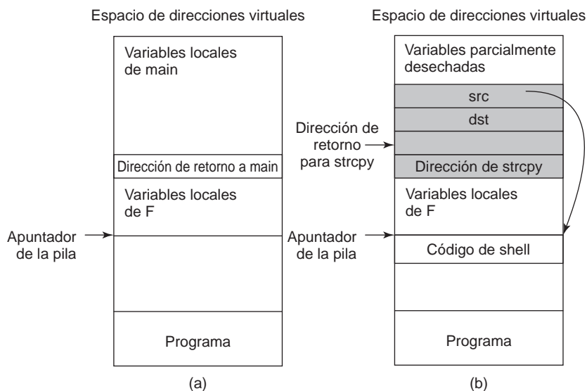
Figura 9-25. (a) La pila antes del ataque. (b) La pila después de que se ha sobrecrito.
