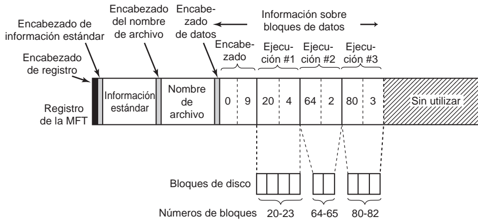
Figura 11-43. Un registro de la MFT para un flujo de tres ejecuciones y nueve bloques.
