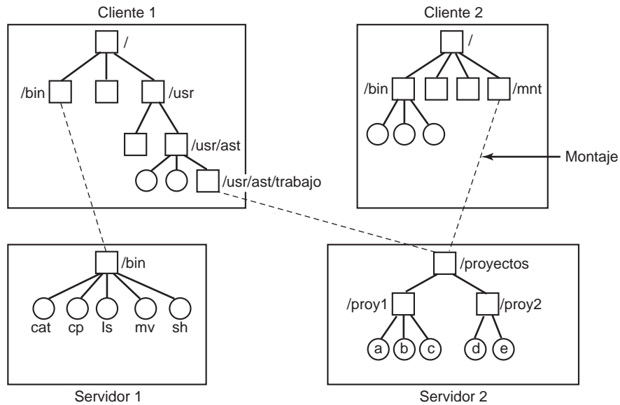
Figura 10-35. Ejemplos del montaje de sistemas de archivos remotos. Los directorios se muestran como cuadros y los archivos como círculos.
