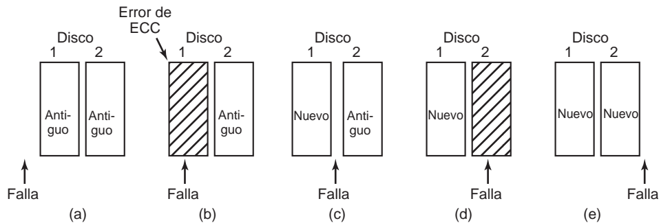
Figura 5-31. Análisis de la influencia de fallos en escrituras estables.
