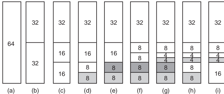
Figura 10-17. Operación del algoritmo de colegas.
