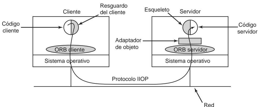
Figura 8-39. Los principales elementos de un sistema distribuido basado en CORBA. Las partes de CORBA se muestran en color gris.
