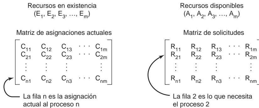
Figura 6-6. Las cuatro estructuras de datos que necesita el algoritmo de detección de interbloques.
