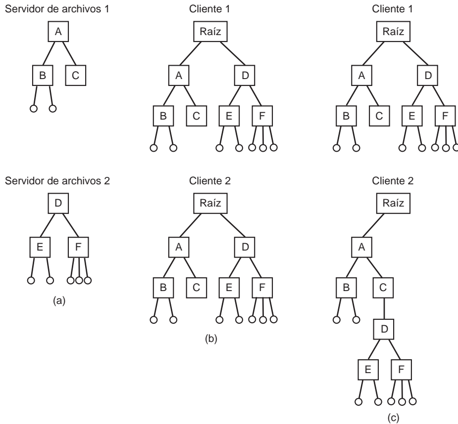
Figura 8-37. (a) Dos servidores de archivos. Los cuadros son directorios y los círculos son archivos. (b) Un sistema en el que todos los clientes tienen la misma vista del sistema de archivos. (c) Un sistema en el que distintos clientes pueden tener distintas vistas del sistema de archivos.
