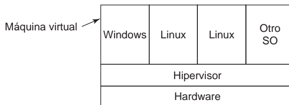
Figura 13-12. Un hipervisor que ejecuta cuatro máquinas virtuales.
