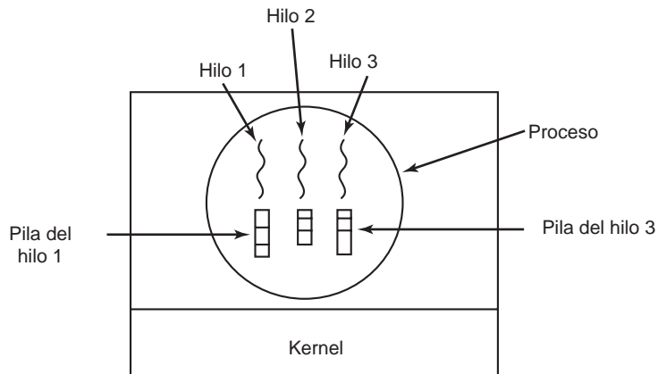
Figura 2-13. Cada hilo tiene su propia pila.
