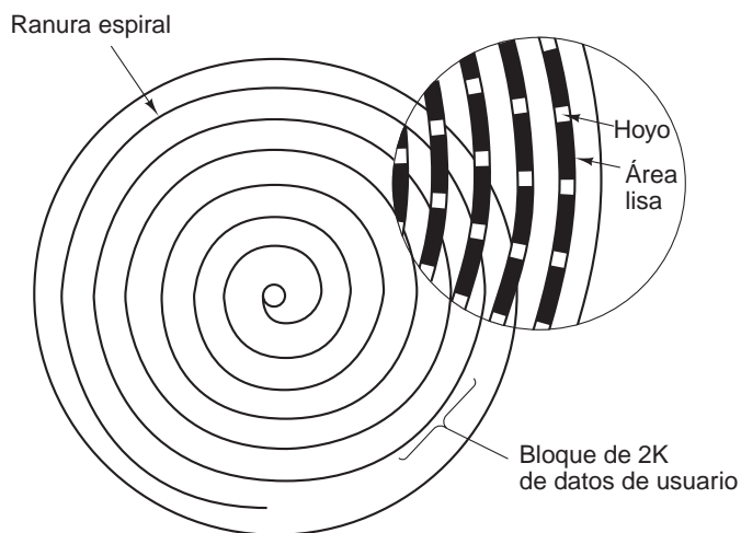
Figura 5-21. Estructura de grabación de un disco compacto o CD-ROM.
