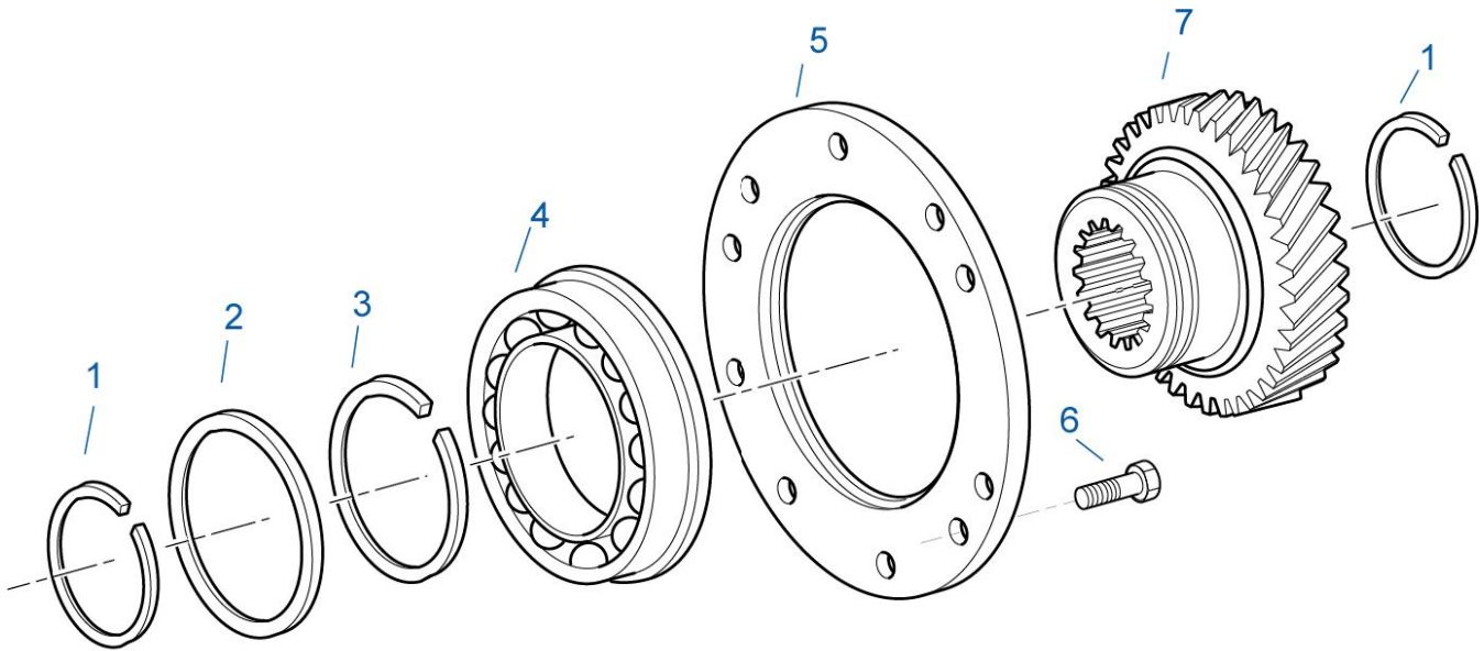
10480-12/92 Aux DG
