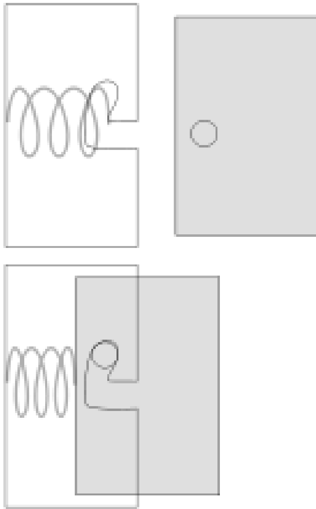
Fig14: Piezas correspondientes que Permite la Conexión Bayoneta.
