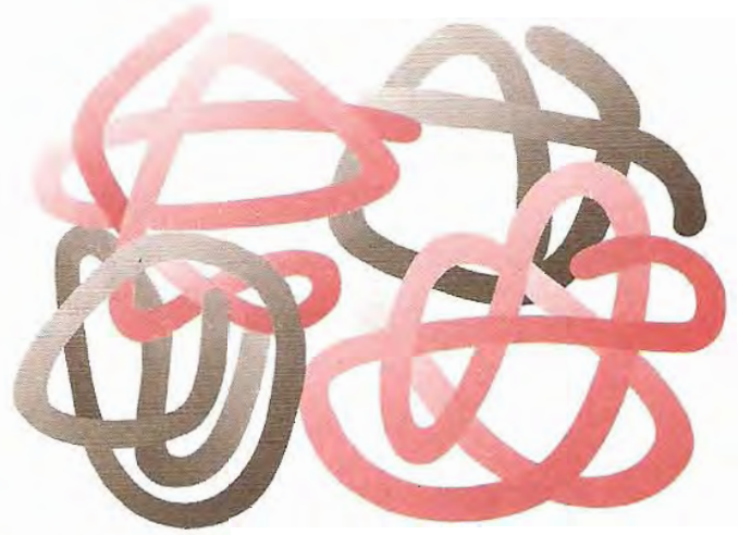
Fig. 3-19. Estructura cuaternaria. Se muestra esquemáticamente la disposición de subunidades polipeptídicas para formar una proteína oligomérica (tetramérica).
