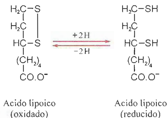
Fig. 22-32. Formas oxidada y reducida de ácido lípico.
