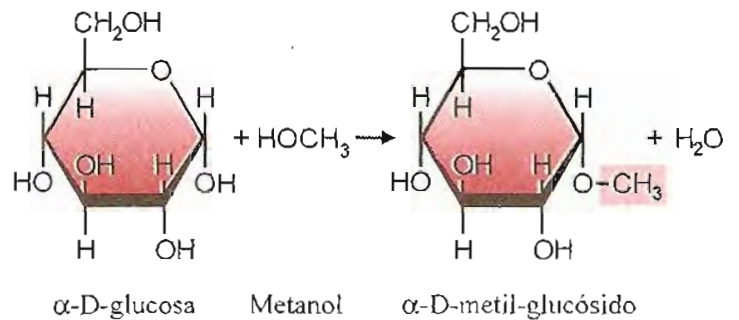
Fig. 4-9. \alpha -D-glucopiranososa (conformación silla C1).
