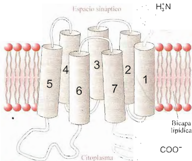
Fig. 24-14. Esquema simplificado de la constitución de un receptor colinérgico muscarínico. Posee siete segmentos transmembranales en hélice (representados como cilindros). Los receptores adrenérgicos, dopaminérgicos, la rodopsina y todos los acoplados a proteínas G tienen una estructura básica similar.
