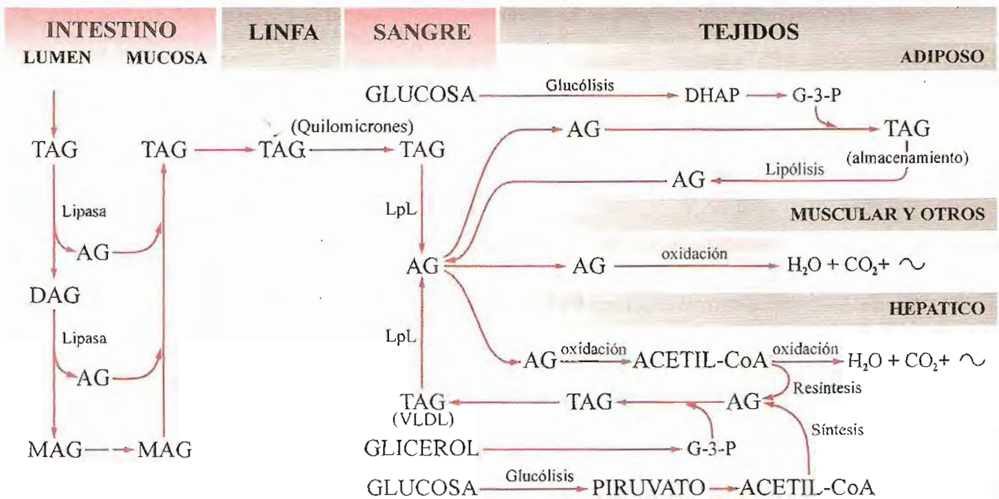
Fig. 14-1. Resumen del metabolismo de triacilglicerol (TAG). DAG: diacilglicerol, MAG: monoacilglicerol, AG: ácidos grasos, DHAP: dihidroxiacetonafofato, G-3-P: glicerol-3-fosfato, LpL: lipoproteína lipasa, VLDL: lipoproteínas de muy baja densidad.
