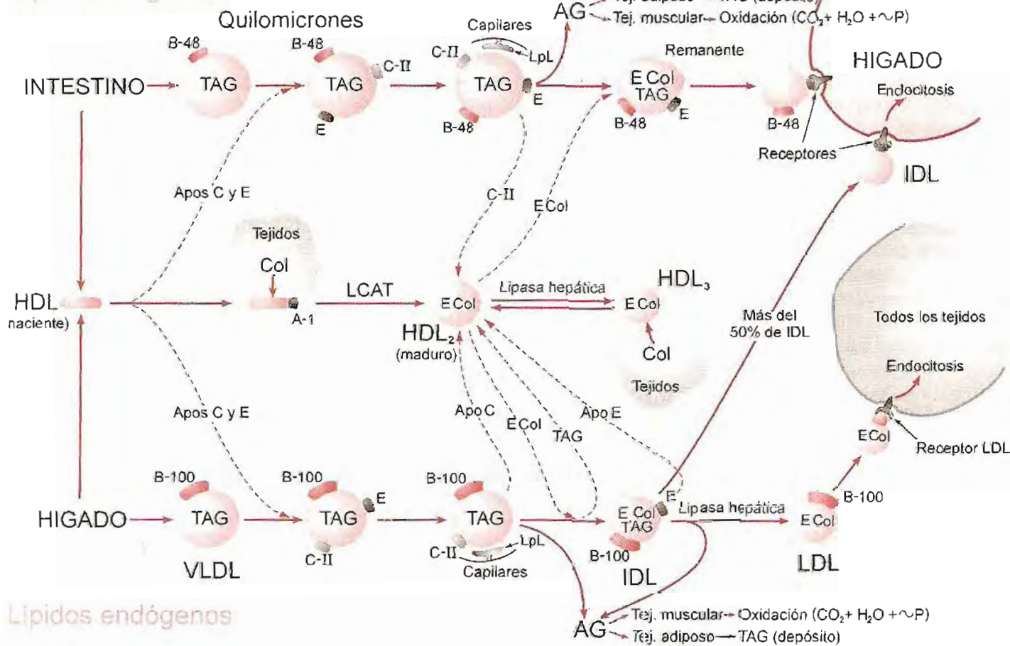
fig. 14-2. Metabolismo de lipoproteínas del plasma. VLDL: lipoproteínas de muy baja densidad, IDL: lipoproteínas de densidad intermedia, LDL: lipoproteínas de baja densidad, HDL: lipoproteínas de alta densidad, TAG: triacilgliceroles, 'col: colesterol libre, ECol: colesterol esterificado, LCAT: lecitina-colesterol aciltransferasa, LpL: lipoproteína lipasa.
