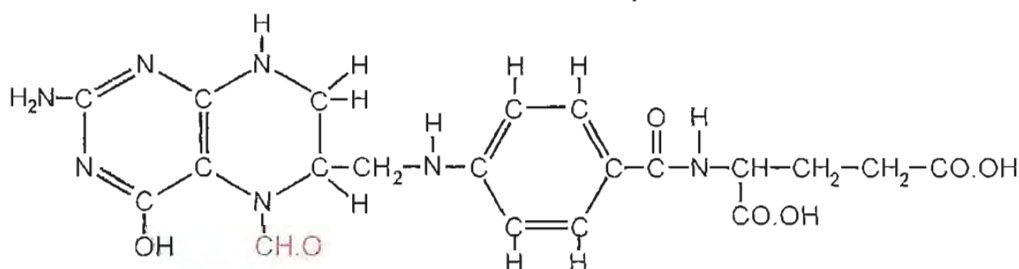
Fig. 22-28. Acido folínico. En rojo se indica el resto formilo.
