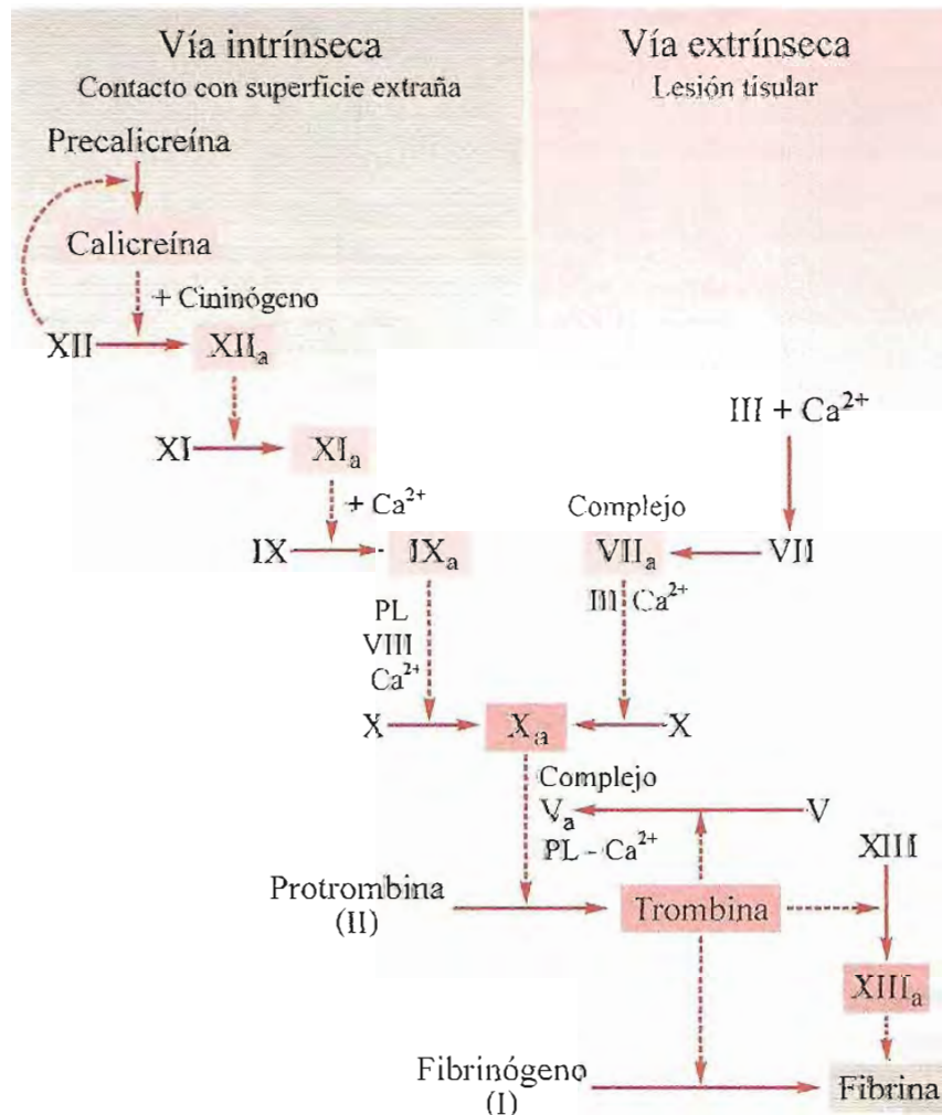
Fig. 24-16. Etapas de la coagulación de la sangre. Las flechas en trazo lleno grueso indican conversión de zimógeno en producto activo. En recuadro las enzimas activadas. Las flechas en trazo cortado señalan acción proteolítica. PL: fosfolípidos.
