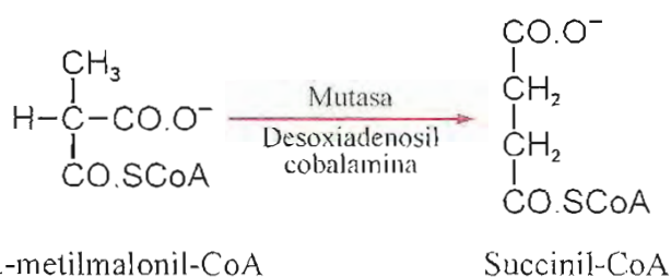
Fig. 22-31. Isomerización de L-metilmaloni-CoA a succinil-CoA.
