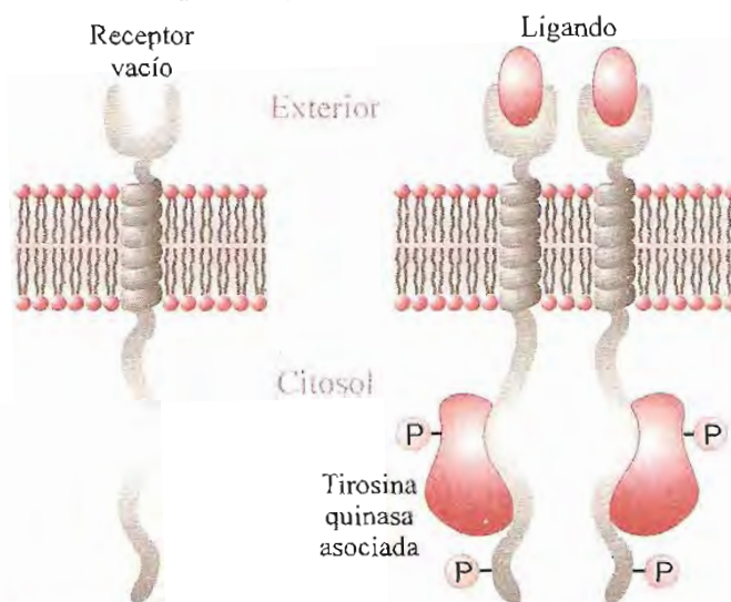
Fig. 21-8. Esquema de un receptor asociado a tirosina quinasa extrínseca. A la izquierda, el receptor inactivo. A la derecha, la unión del ligando (hormona de crecimiento, citoquina) induce la dimerización del receptor y modifica el dominio citosólico de manera que puede interactuar y activar una tirosina quinasa, la cual fosforila restos de tirosina en la propia enzima y en el receptor.
