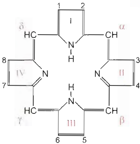
Fig. 3-25. Núcleo porfina. Los núcleos pirrolo se indican con números romanos; los puentes metino, con letras griegas. Los números 1 a 8, posiciones que pueden ser sustituidas por diferentes cadenas carbonadas.
