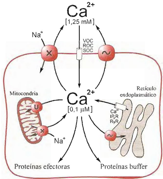
Fig. 23-12. Regulación del calcio intracelular. ~ : Ca^{2+} -ATPasa; x: intercambiador Na^+/Ca^{2+} ; U: uniporter ; IP_3R : receptor de inositol-1,4,5-trisfosfato; RyR: receptor de rianodina.
