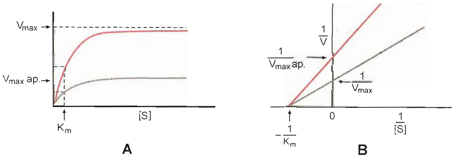
Fig. 8-10. Efecto de la presencia de un inhibidor no competitivo sobre la actividad enzimática (línea roja: sin inhibidor; línea gris: con inhibidor). A. Curva de velocidad inicial en función de la concentración de sustrato. B. Representación de dobles recíprocas.
