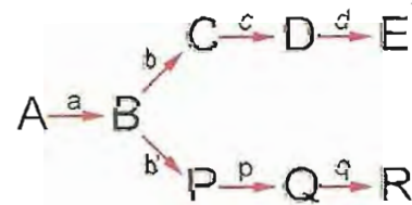
Fig. 12-2. Ramificación en una secuencia de reacciones.
