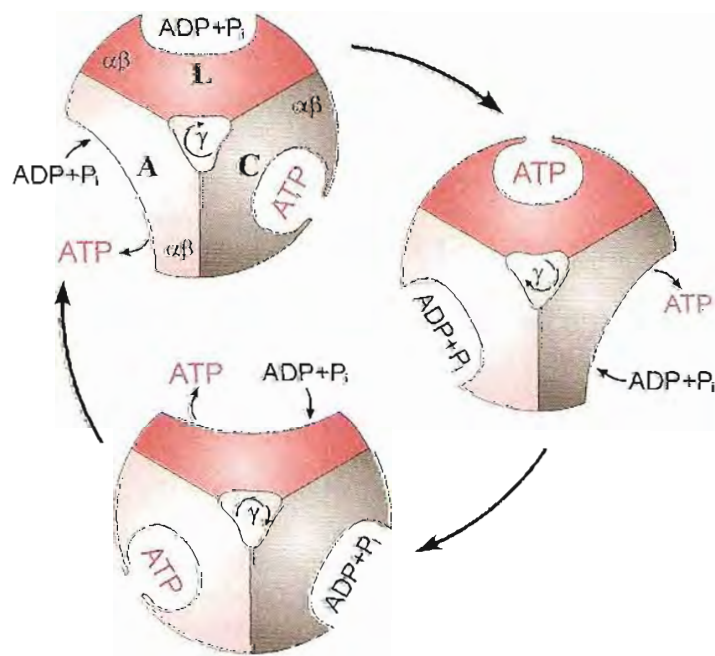
Fig. 9-17. ATP sintasa como máquina rotatoria para la síntesis de ATP. Corte transversal (muy esquemático). La rotación de la subunidad γ determina que el sitio catalítico en cada subunidad β del complejo F 1 pase sucesivamente por tres conformaciones: laxa (L), cerrada (C) y abierta (A). En un giro completo se liberan tres moléculas de ATP.
