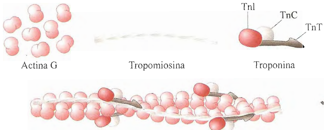
Fig. 24-7. En la parte superior de la figura se representan las proteínas constituyentes de los filamentos delgados; abajo se ilustra el ensamble de un filamento fino. Los monómeros de actina G se disponen formando una hebra o cadena de actina F, que semeja una doble hélice. Las moléculas de tropomiosina se alojan en los surcos helicoidales que forma la hebra de actina. La troponina, constituida por tres proteínas (TnT, TnI y TnC), se fija al filamento de tropomiosina a intervalos regulares.
