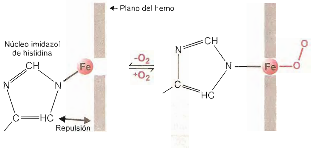
Fig. 3-31. Cambio de posición del Fe^{2+} del hemo durante la oxigenación de Hb. En Hb desoxigenada (izquierda), el átomo de hierro está fuera del plano formado por el hemo porque el anillo imidazol de la histidina a la cual el Fe^{2+} está unido es rechazada por un N del hemo. Cuando la Hb se oxigena (derecha), el Fe^{2+} es desplazado hacia el plano del hemo y arrastra tras sí a la histidina, con las consiguientes modificaciones en la conformación de la cadena a la cual el aminoácido pertenece.
