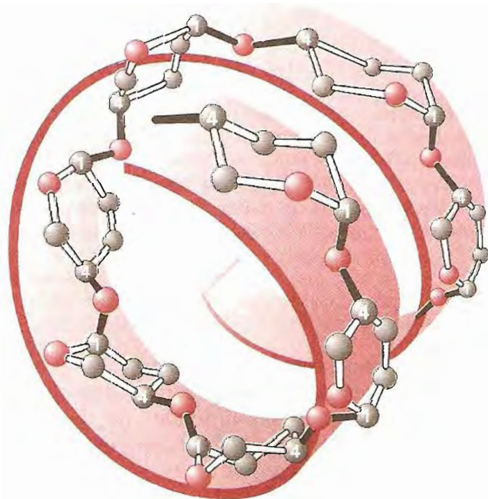
Fig. 4-13. Conformación helicoidal de la amilosa. Modelo de esferas y varillas. Sólo se representan los elementos del anillo pirano. En negro C1 a 5, en rojo: oxígeno del ciclo y de la unión glucosídica \alpha -1 \rightarrow 4.
