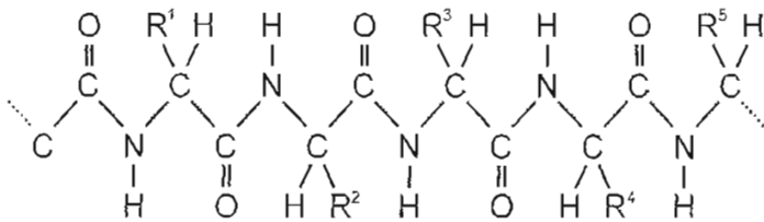
Fig. 3-11. Representación simplificada de un trozo de polipéptido. R¹, R², R³, etc., indican las cadenas laterales de residuos aminoácidos.
