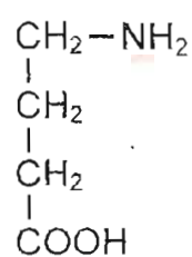
Ácido \gamma -aminobutírico
