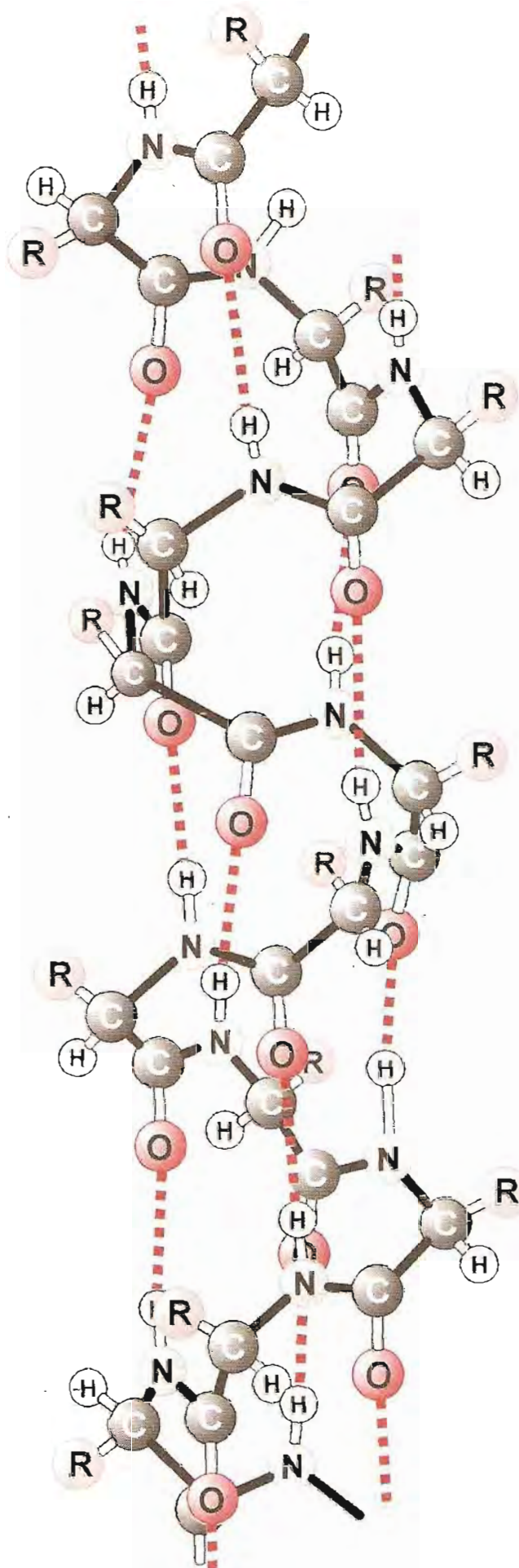
Fig. 3-15. Modelo molecular con esferas y varillas de una hélice \alpha . R representa cadenas laterales de los restos aminoacídicos. Las líneas de puntos rojos indican los puentes de hidrógeno que estabilizan la hélice (imitado de Corey y Pauling).
