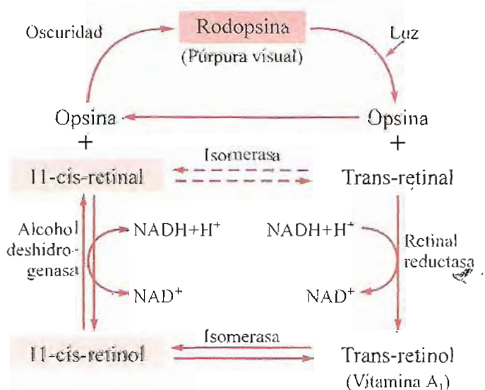
Fig. 22-5. Ciclo de la rodopsina.
