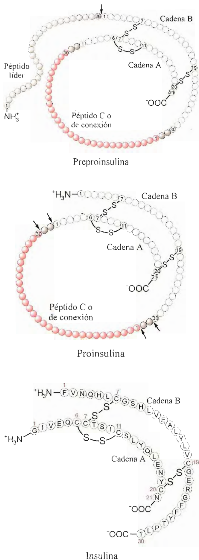
Fig. 21-35. Esquema de las moléculas de preproinsulina, proinsulina e insulina. En esta última se indican los aminoácidos constituyentes de la insulina humana.
