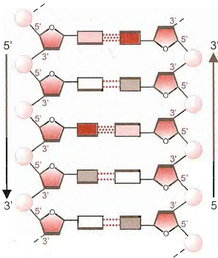
Fig. 6-10. Esquema de un segmento de molécula de ADN en el cual se muestra el apareamiento de las cadenas en la doble hélice. Nótase cómo la orientación de las uniones de fosfatos (esferas rosadas) en una de las cadenas tiene un sentido opuesto al de la otra. Las líneas de puntos rojos representan los enlaces tipo puente de hidrógeno que mantienen apareadas las bases, indicadas como rectángulos: guanina: rosa, citosina: rojo, adenina: blanco y timina: gris.
