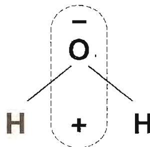
Fig. 2-3. Distribución de las cargas eléctricas en la molécula de agua.
