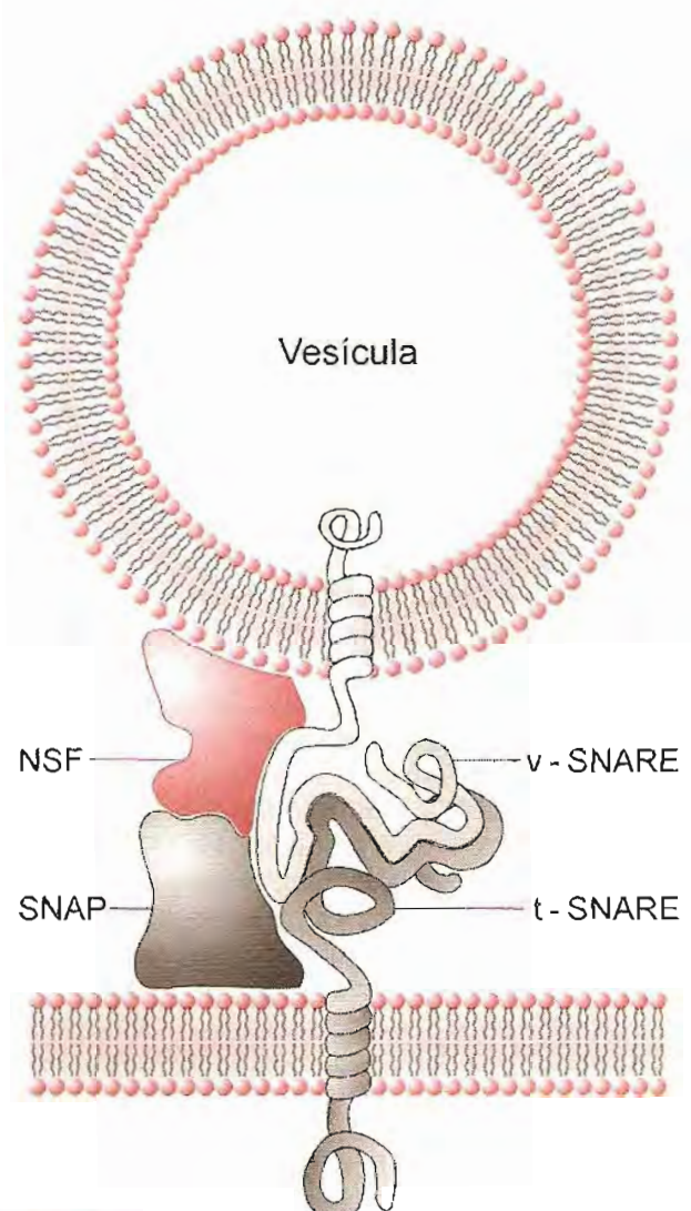
Fig. 10-20. La vesícula reconoce su destino en la membrana “blanco”, por la interacción entre el par v - SNARE y t - SNARE . El complejo de SNARE s une las proteínas NSF y SNAP que promueven la fusión de las membranas.
