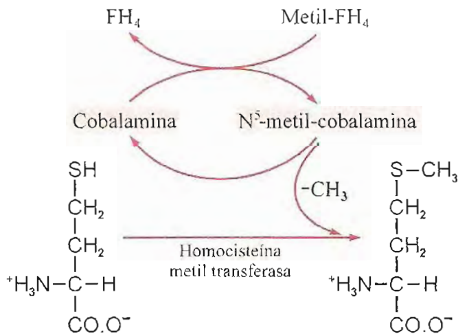
Fig. 22-30. Participación de vitamina B 12 en la reacción de conversión de homocisteína en metionina.
