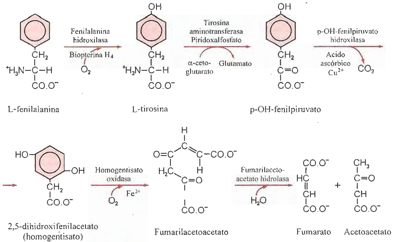
Fig. 15-9. Vía catabólica de fenilalanina y tirosina.
