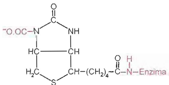
Fig. 22-26. Complejo \text{CO}_2 -biotina-apoenzima (" \text{CO}_2 activado").
