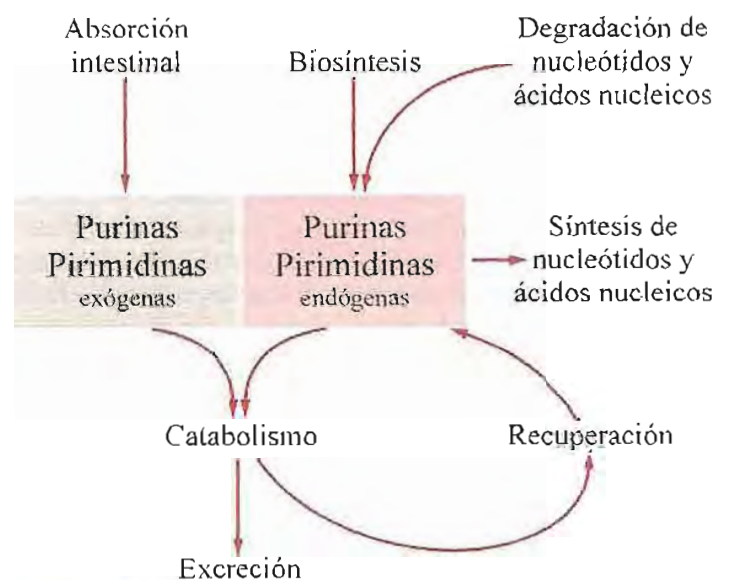
Fig. 17-1. Resumen del metabolismo de bases púricas y pirimídicas.
