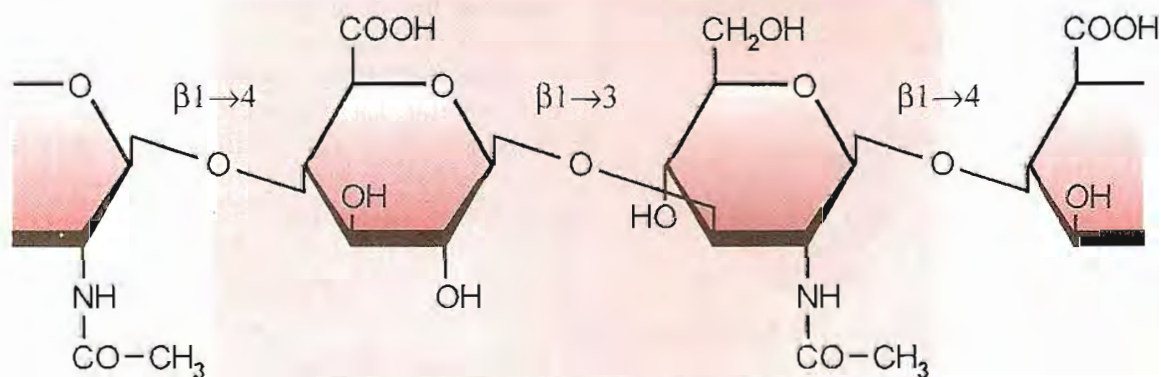
Fig. 4-17. Unidad estructural de ácido hialurónico (disacárido sobre rectángulo rosado). Acido D-glucurónico- \beta -1 \rightarrow 3-N-acetil-D-glucosamina. Al pH del organismo, la función carboxilo está disociada ( -\text{COO}^- ).
