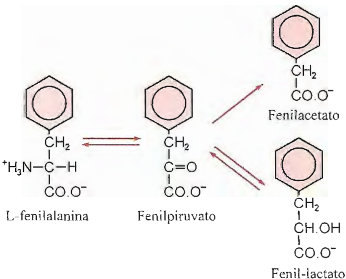
Fig. 15-10. Vía metabólica alternativa de fenilalanina.
