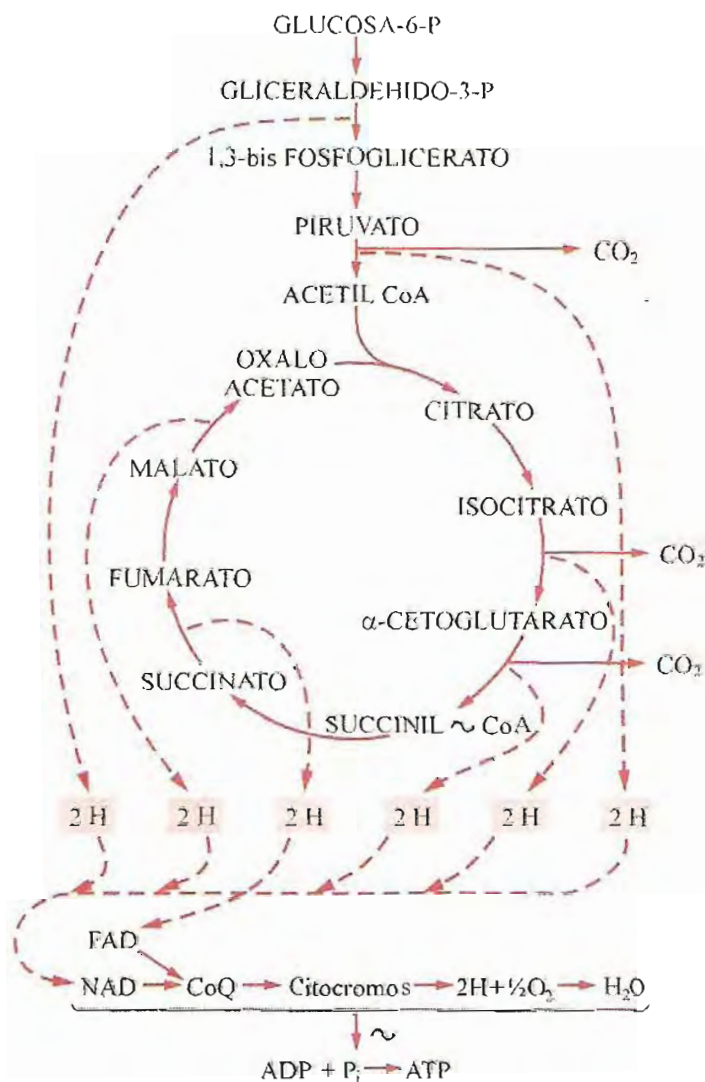
Fig. 13-9. Esquema del catabolismo oxidativo de la glucosa.
