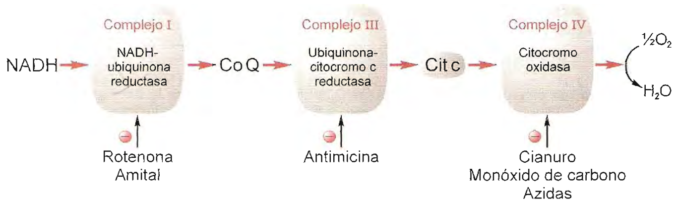
Fig. 9-12. Cadena respiratoria. Sitios de bloqueo por inhibidores.
